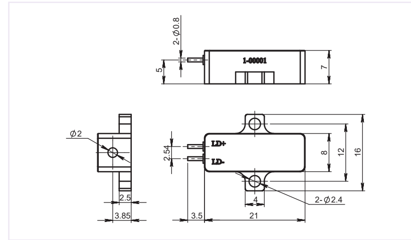
CL-LF100-B, CL-LF200-B
