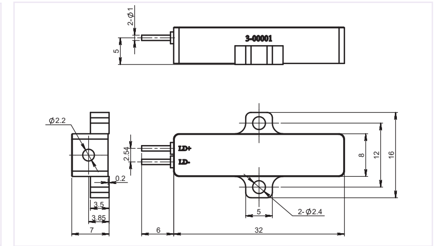
CL-LF400-B, CL-LF500-B
