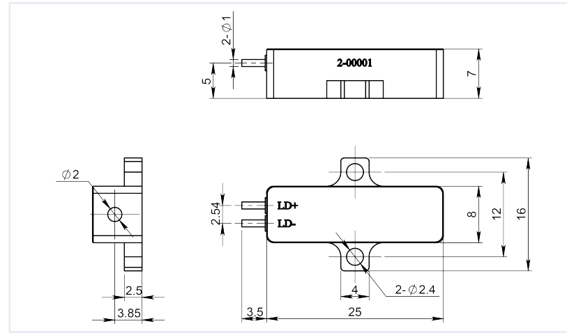
CL-LF300-B
