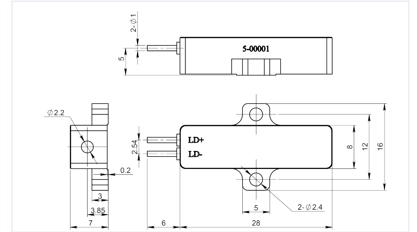
CL-LF400-B
