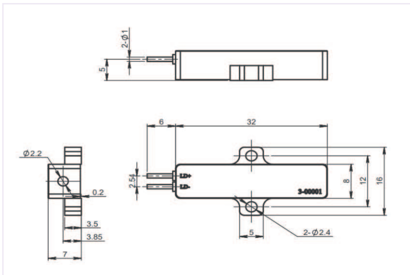
CL-LF500-B
