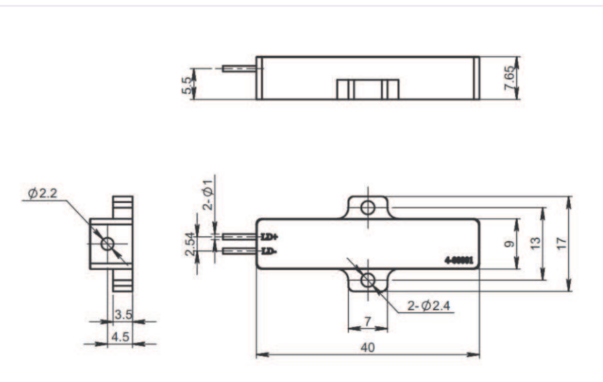
CL-LF800-B, CL-LF1000-B
